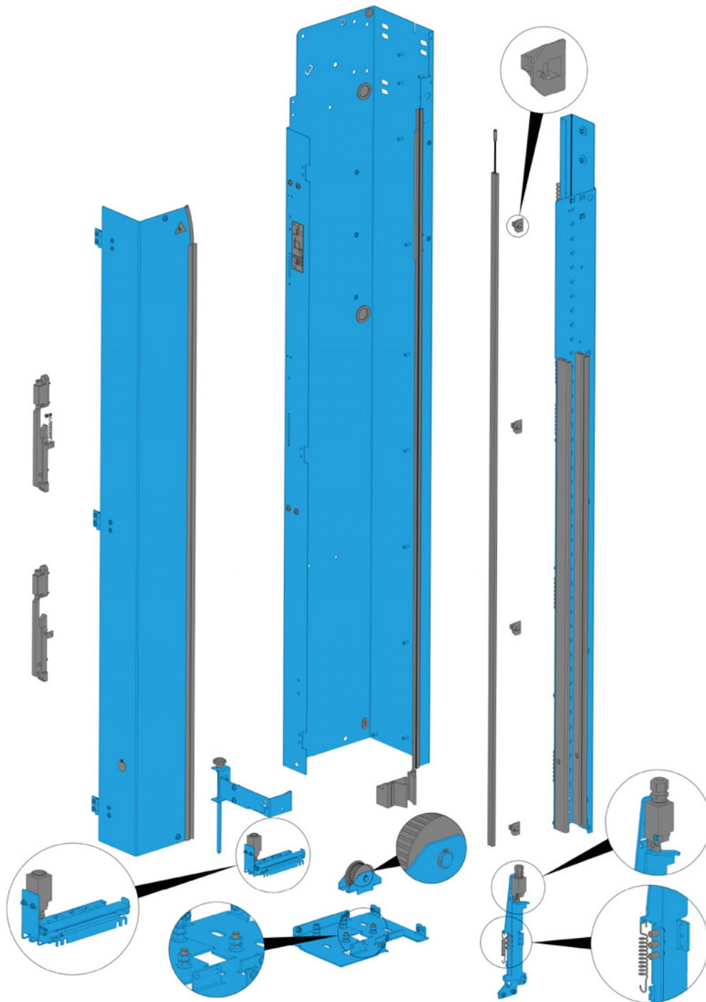
Fig. 70: Left side frame
