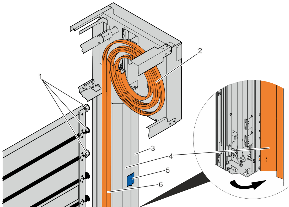
Fig. 23: Door leaf guide
